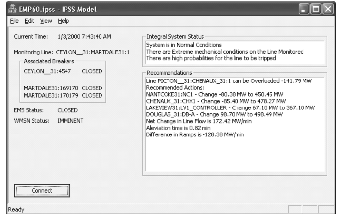
Fig. 3. IPSS output.
