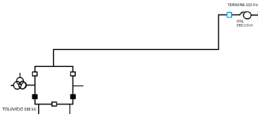
Figura 6. Diagrama de subestaciones Tolviejo y Ternera 110 KV.
