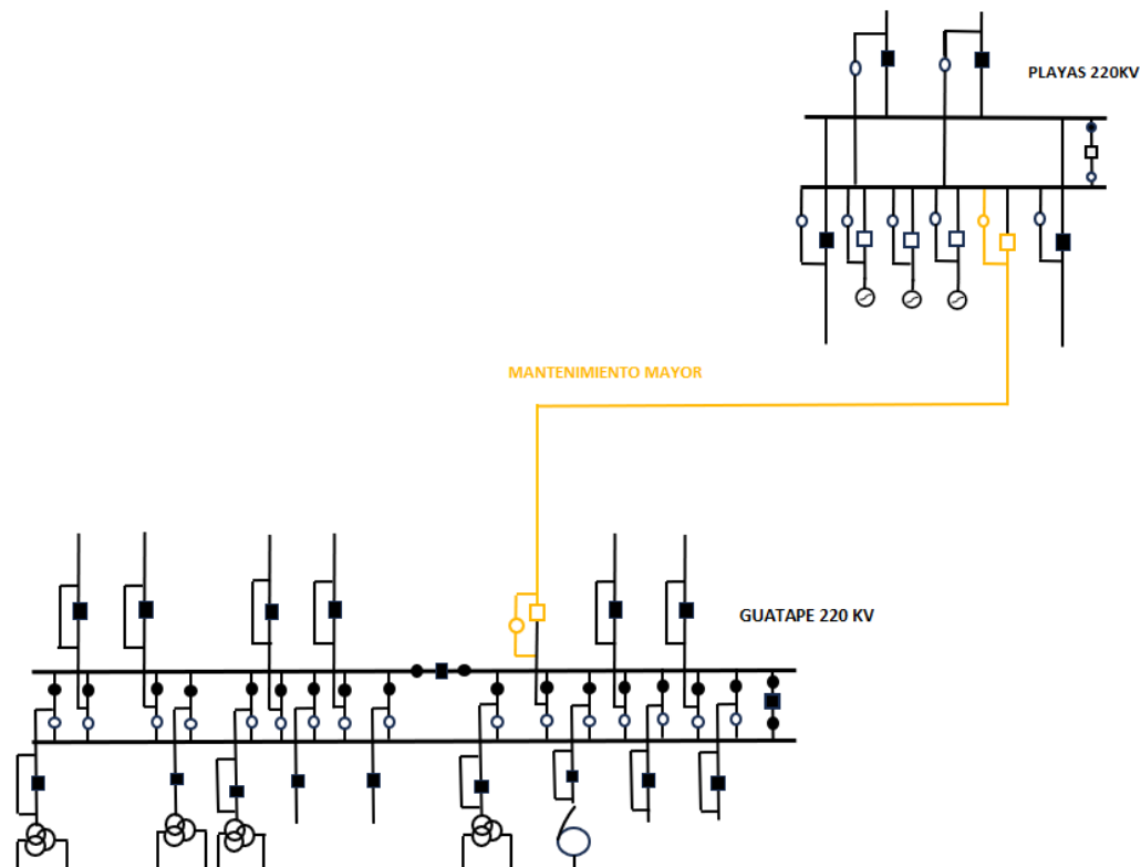
Figura 18. Diagrama de las subestaciones Guatapé y Playas 220 KV
