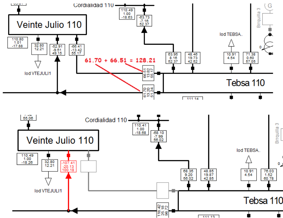
Figura 5. Ejemplo cálculo de Corte
