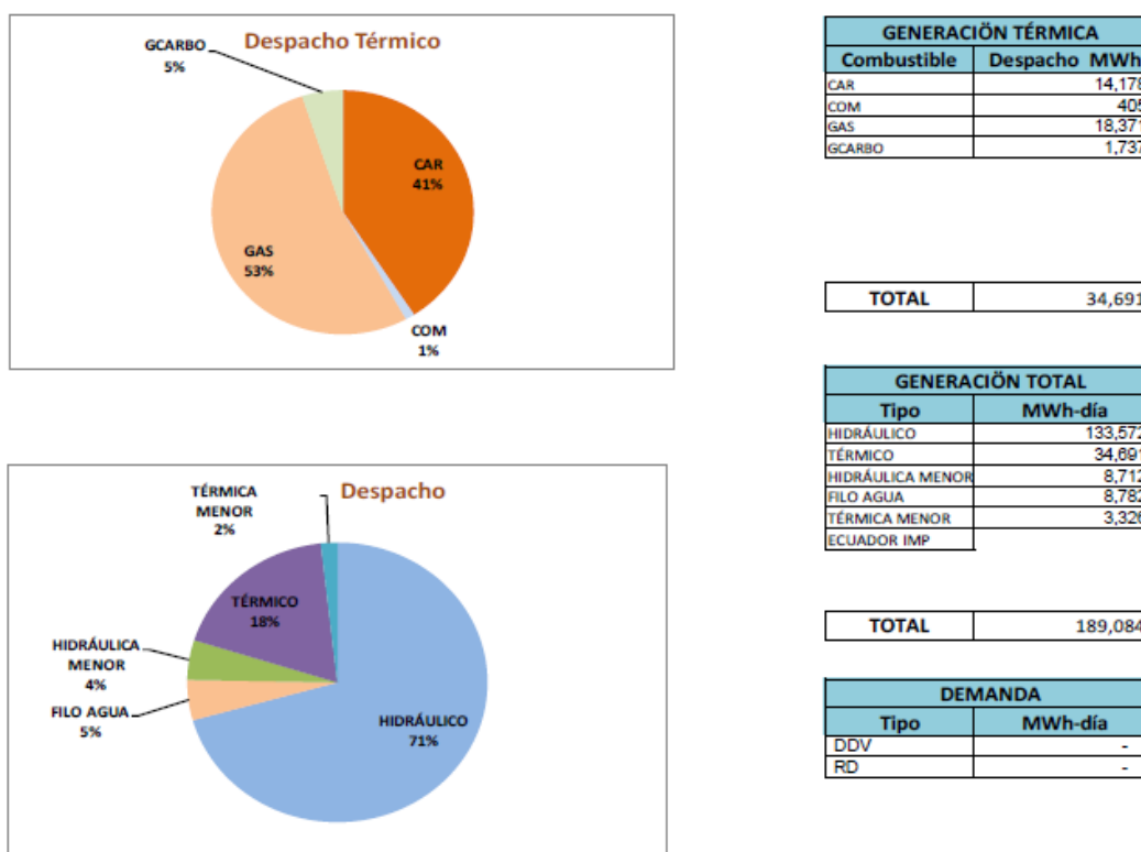
Figura 2. Perfil de Generación
